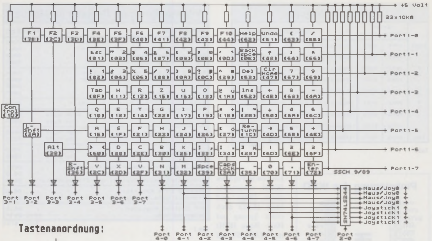
Abb. 2: IKBD-Tastaturmatrix
