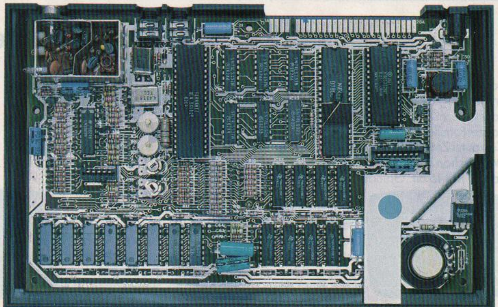
Innenleben des Spectrum, 48 KByte-Version (untere Chip-Reihe: RAMs)
