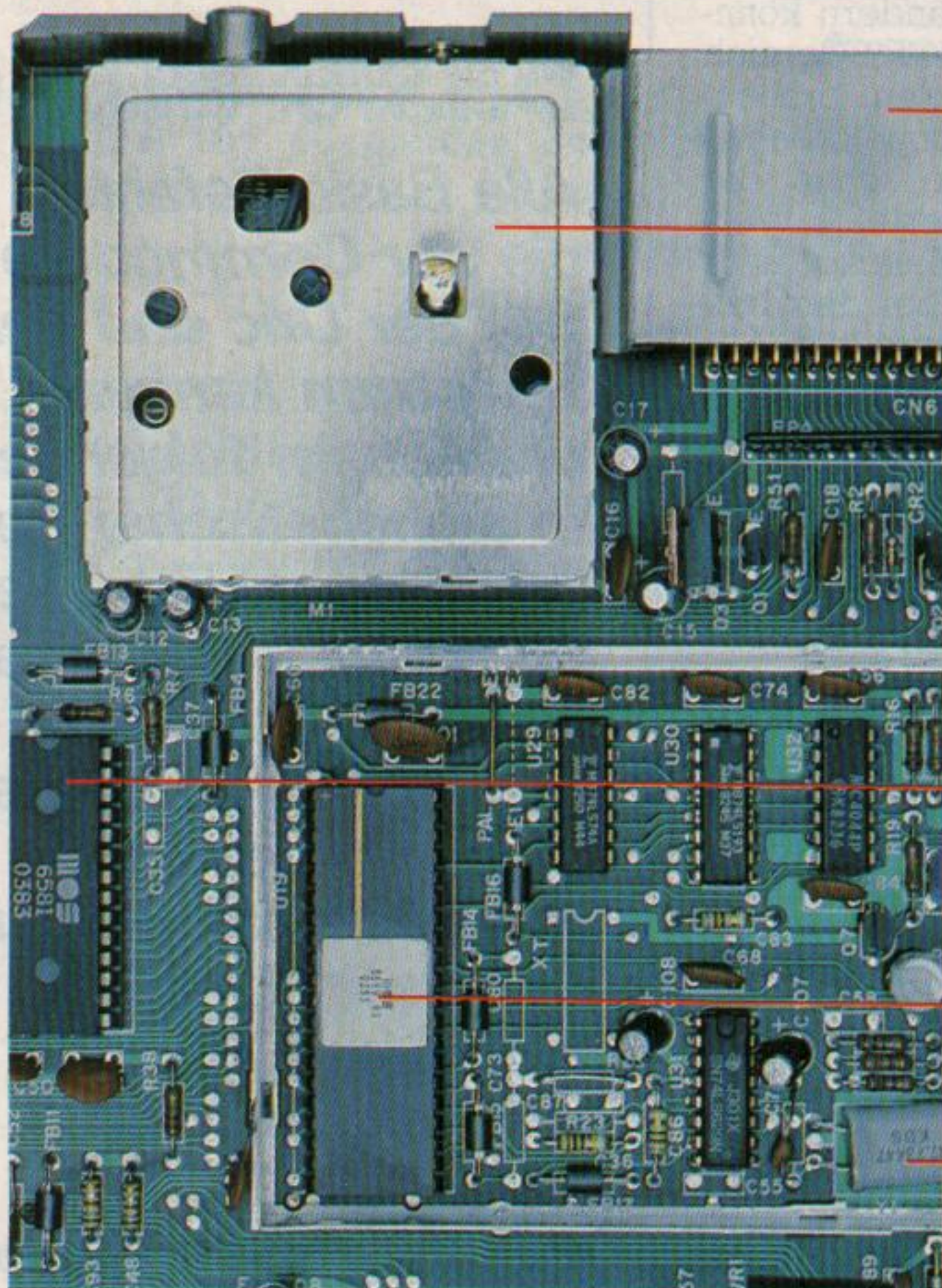
Bildteil des Commodore 64
