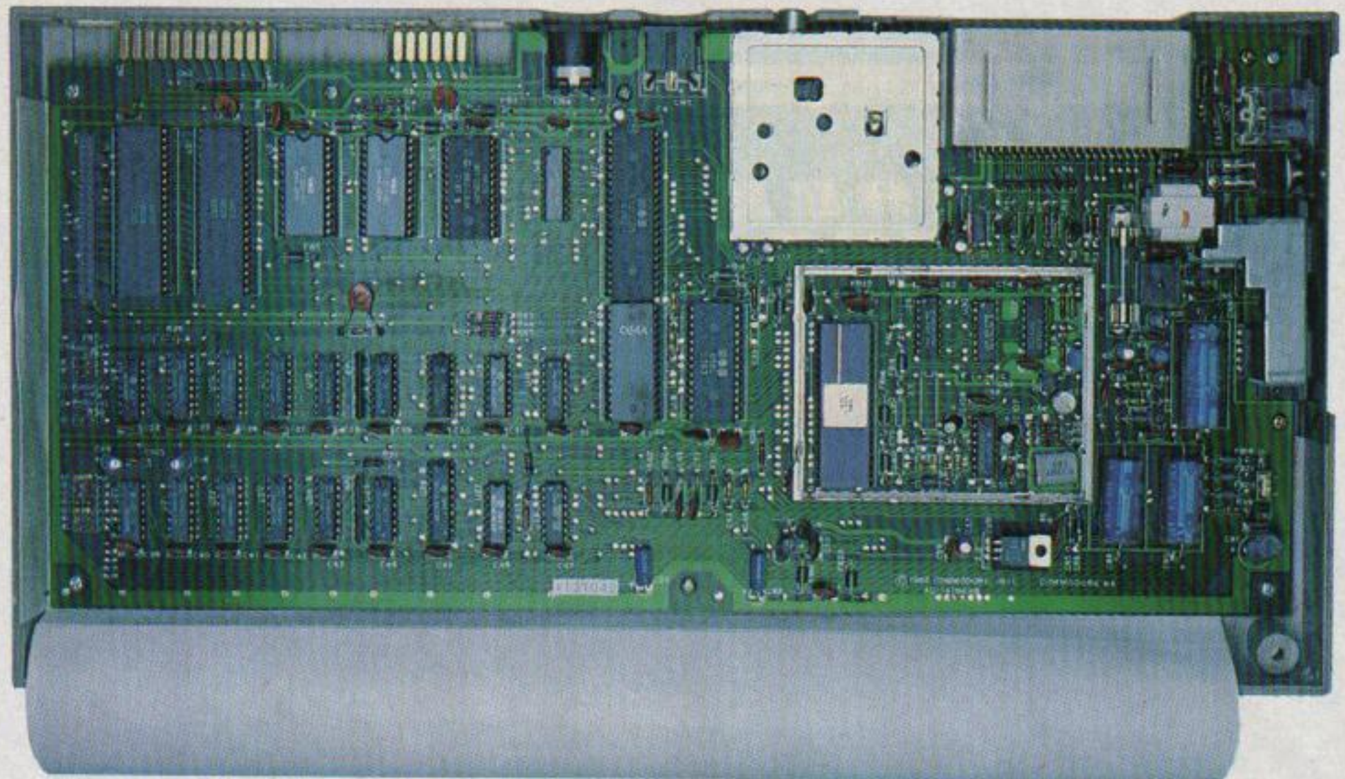
Innenleben des Commodore 64 (linke Hälfte: CPU und RAMs)
