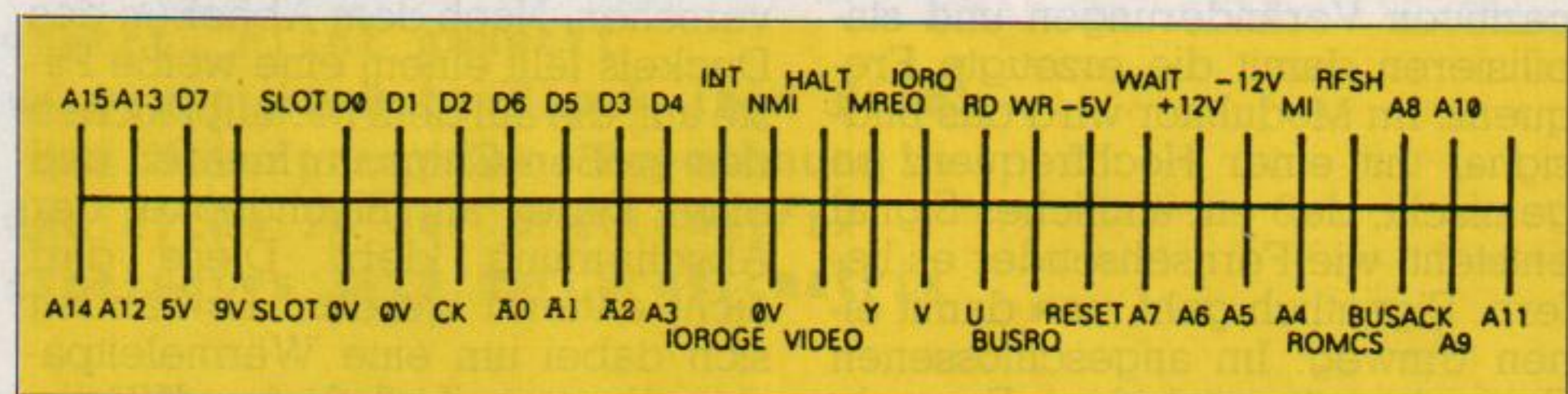
Bus-Erweiterung beim Spectrum
