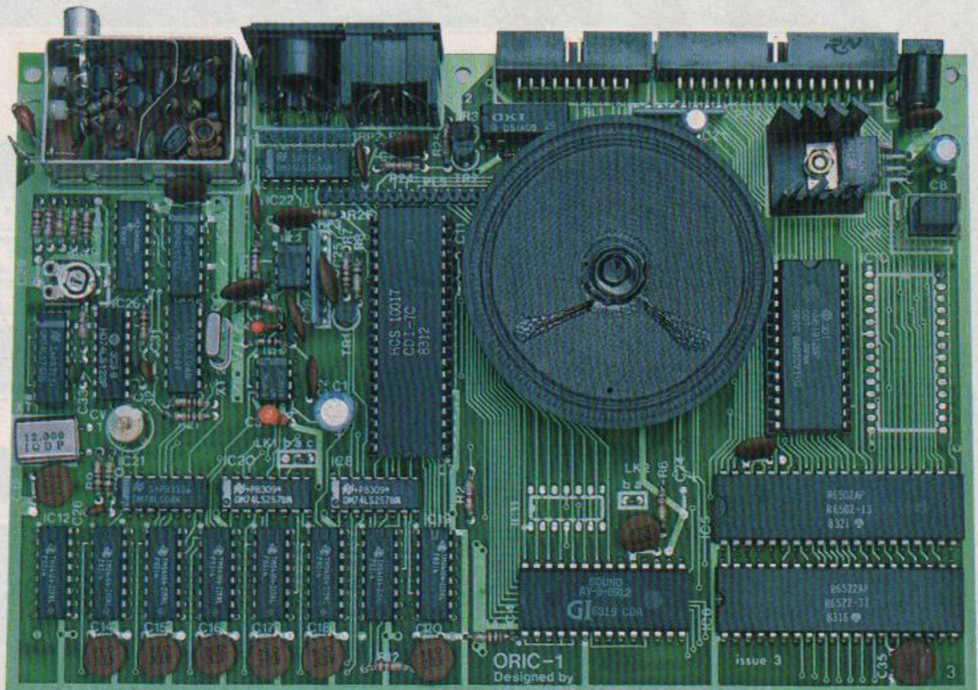
Innenleben des Oric-1 (im Original etwa halb so groß wie der Commodore)
