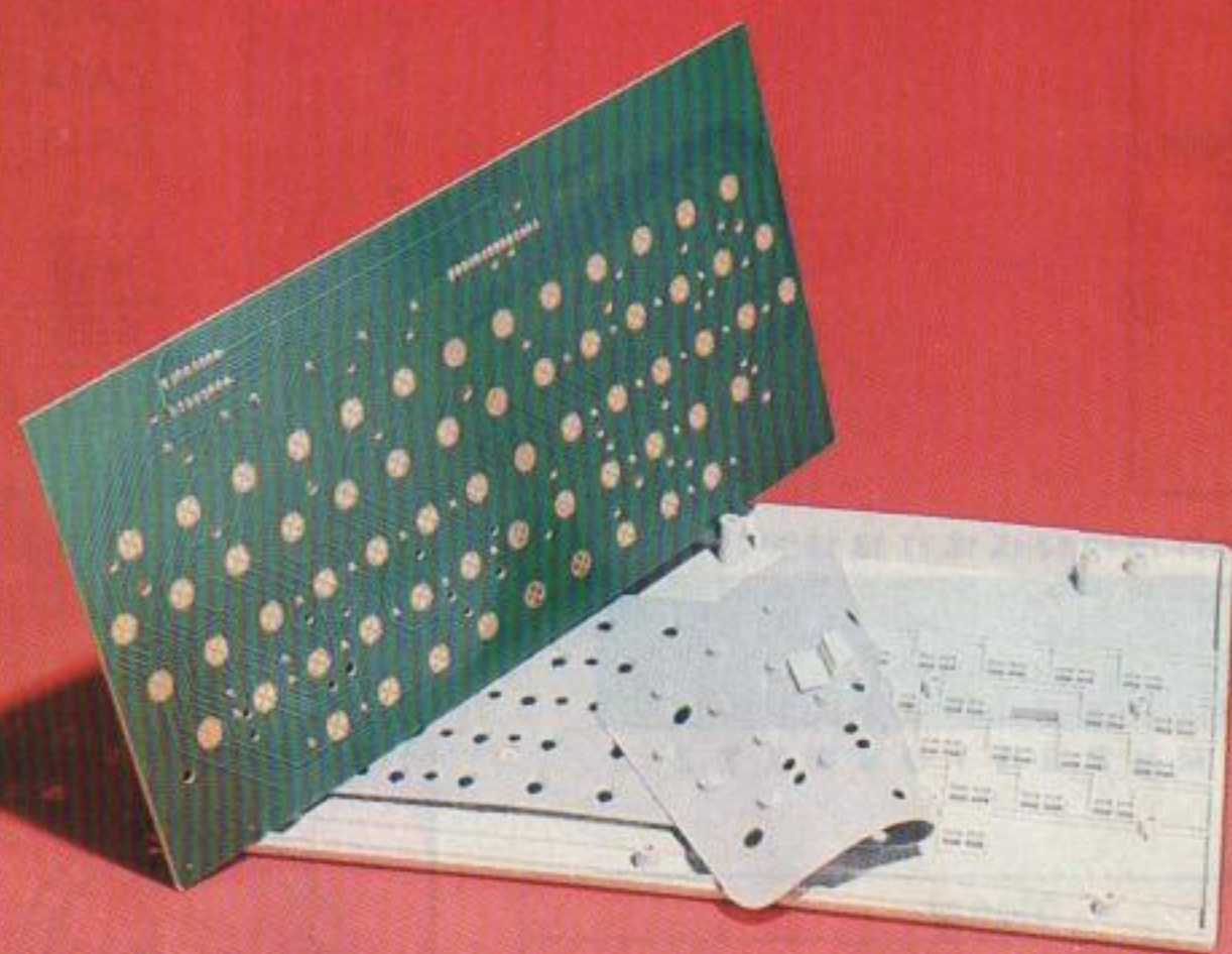
Oric-1: Tastaturplatte, Gummimatte und Hartplastiktasten
