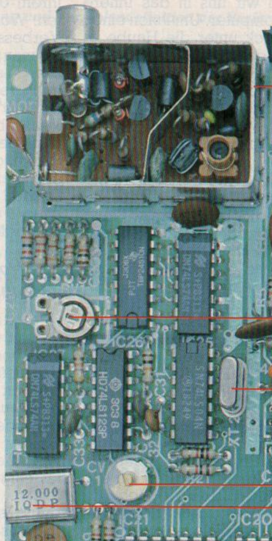
Bildteil des Oric-1
